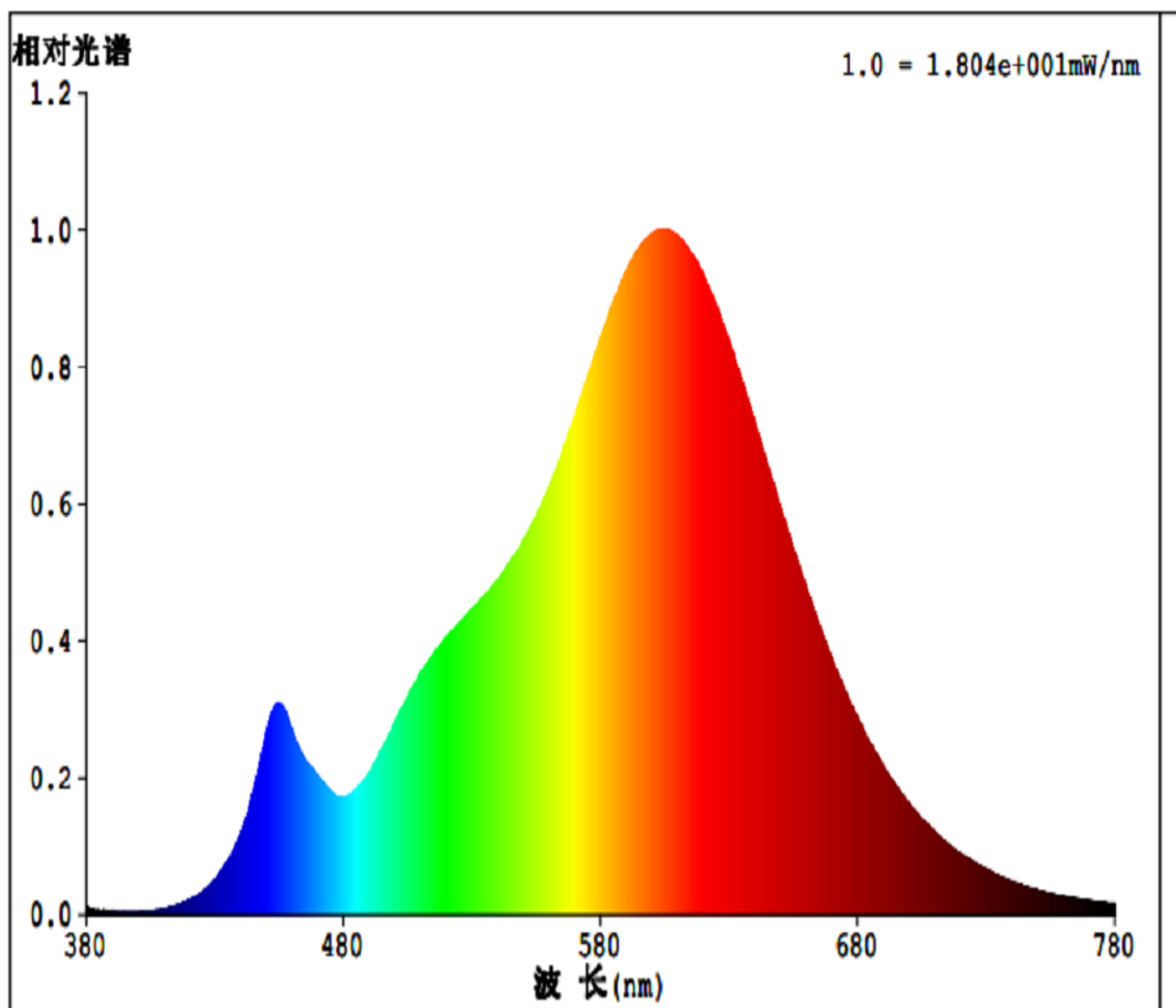
光谱分布
